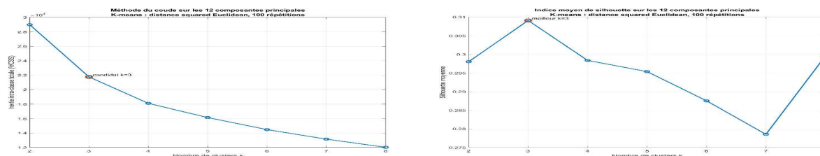
Figure 2. Détermination du nombre de zones par la méthode du coude et l'indice de silhouette.
