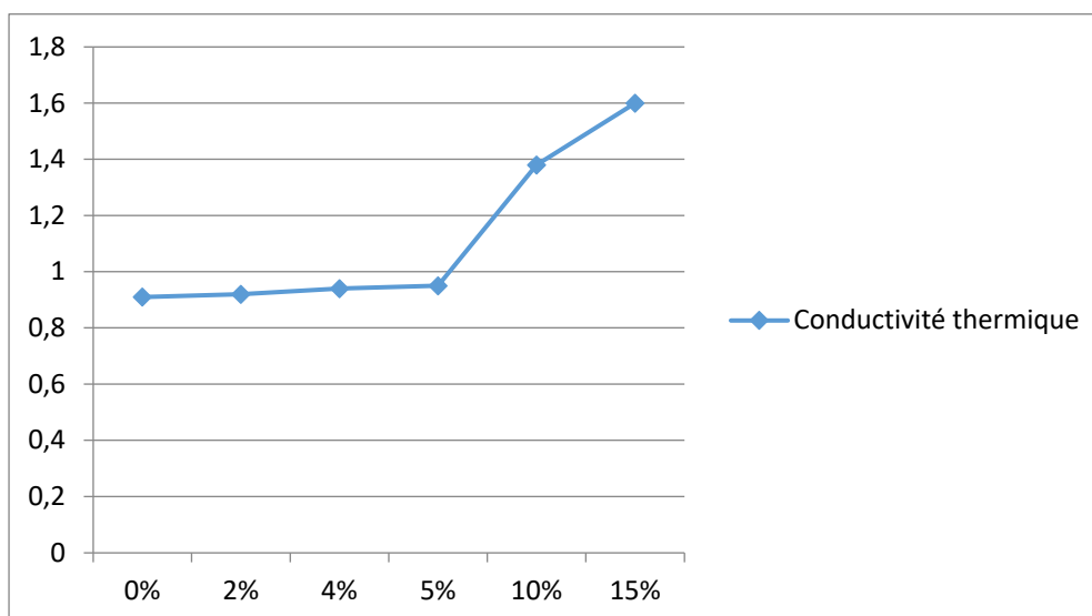
Figure 4 : la valeur de la conductivité thermique en fonction de la teneur en ciment
