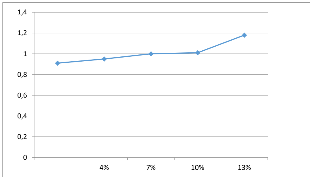
Fig 9: valeur de la conductivité thermique en fonction de la teneur en chaux
