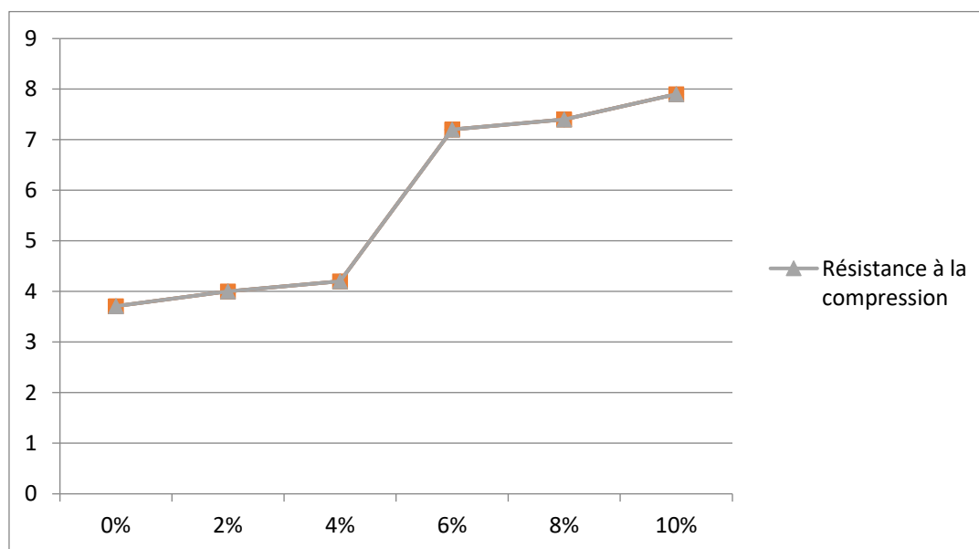
Figure n°1 : Résistance à la compression en fonction de la teneur en ciment
