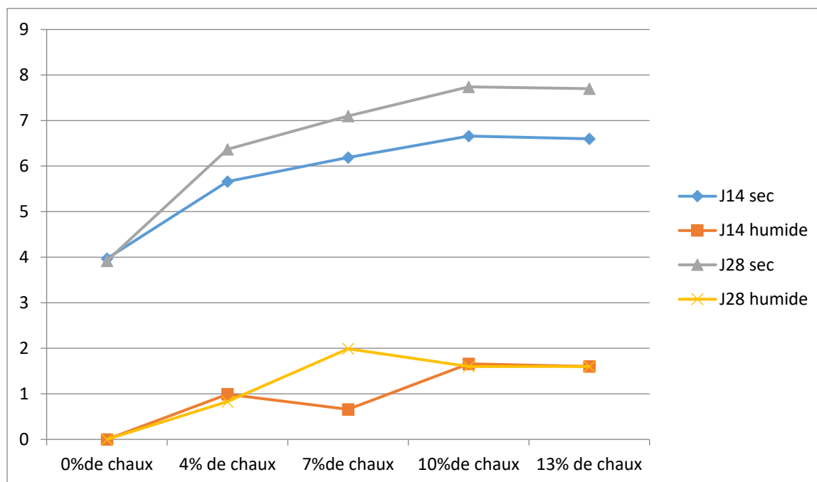
Figure 8: Résistance à la compression en fonction de la teneur en chaux (pourcentage en masse)
