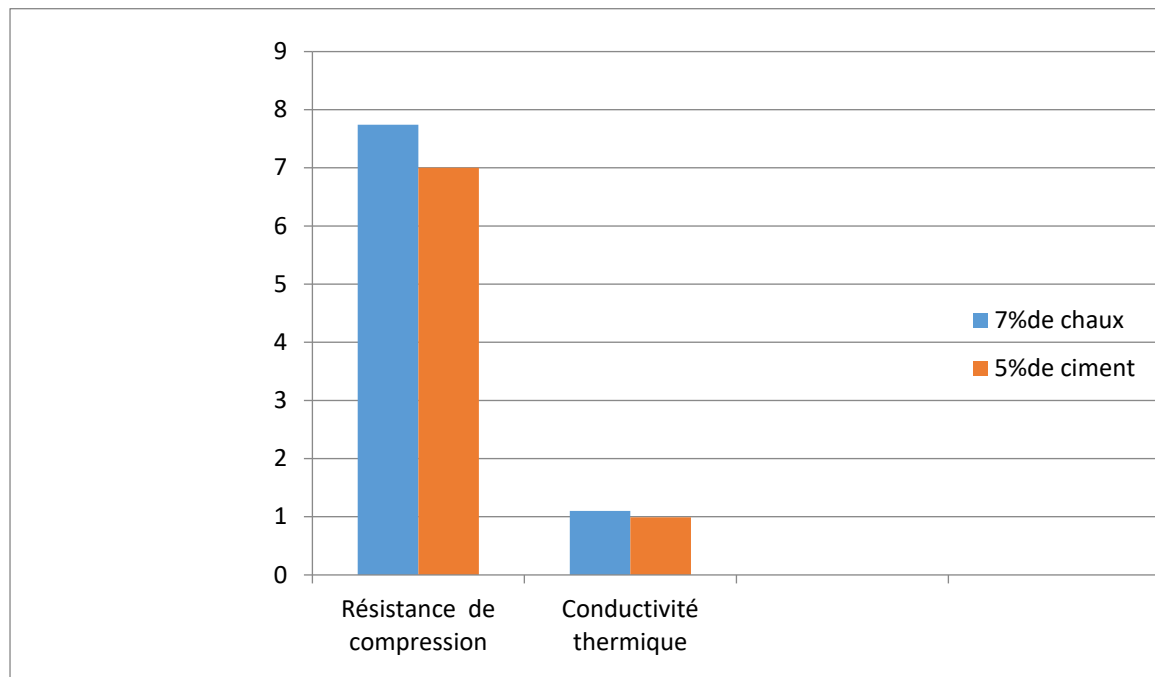
Figure 10 : Comparaison des résultats de la stabilisation au ciment et à la chaux
