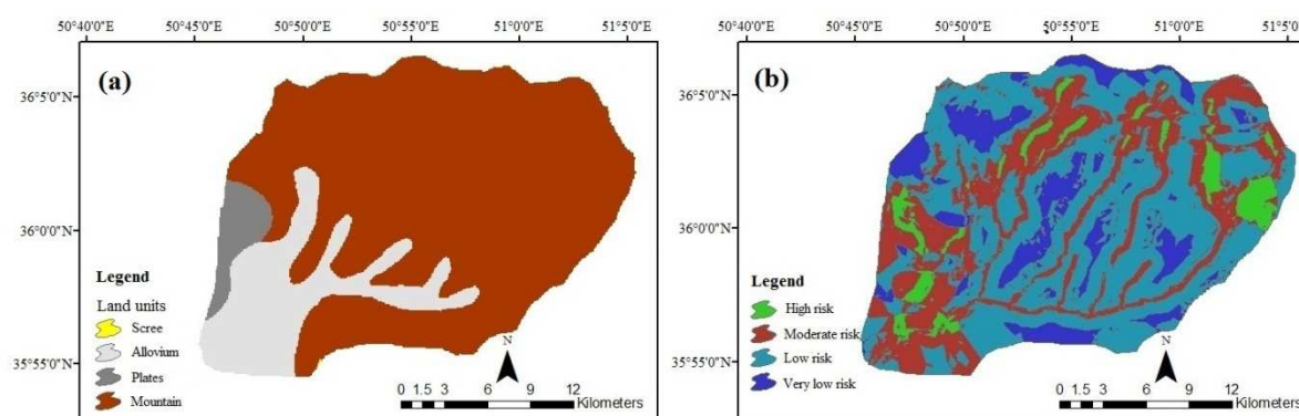
Fig. 13. a) Land unit, b) The landslide hazard zonation map.
