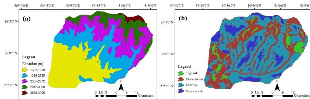
Fig. 17. a) Elevation map. b) The landslide hazard zonation map
