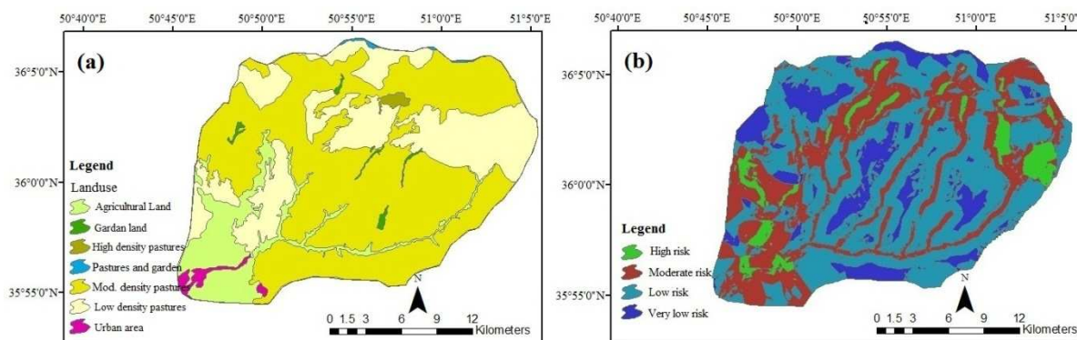
Fig. 10. a) Landuse map, b) The landslide hazard zonation map
