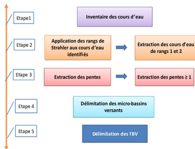
Fig.2. Synthèse des méthodes d'inventaire et de délimitation des têtes de bassin de la Mékrou
