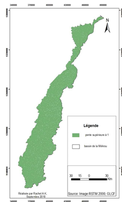
Fig.7. Pentes supérieures ou égales à \geq 1
