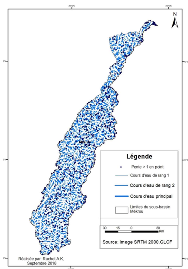
Fig.9. Superposition des Pentes supérieures ou égales à \geq 1 avec les cours d'eau de rangs 1 et 2
